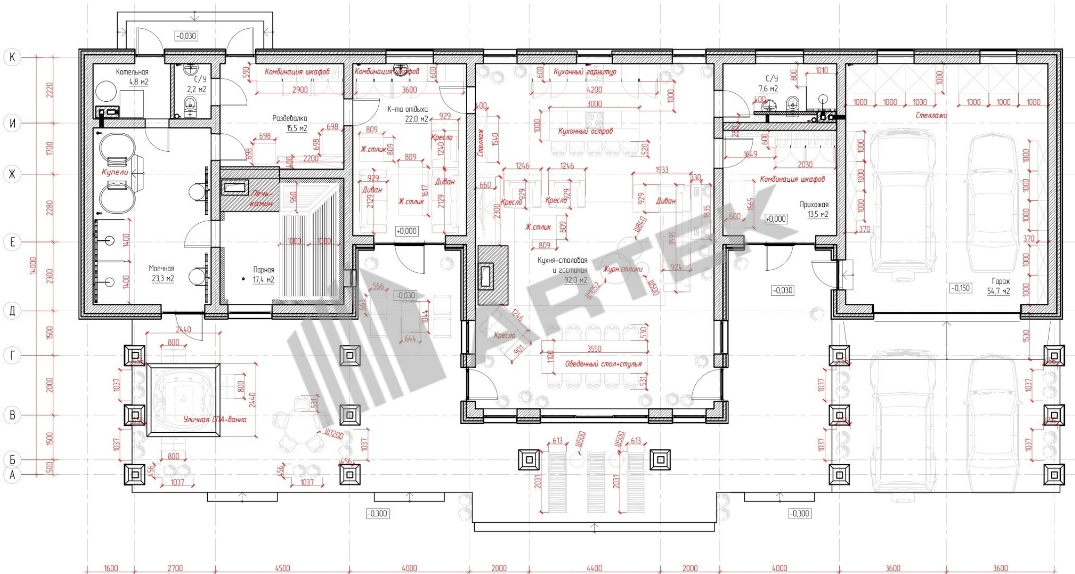
План расстановки мебели и оборудования М 1:100
