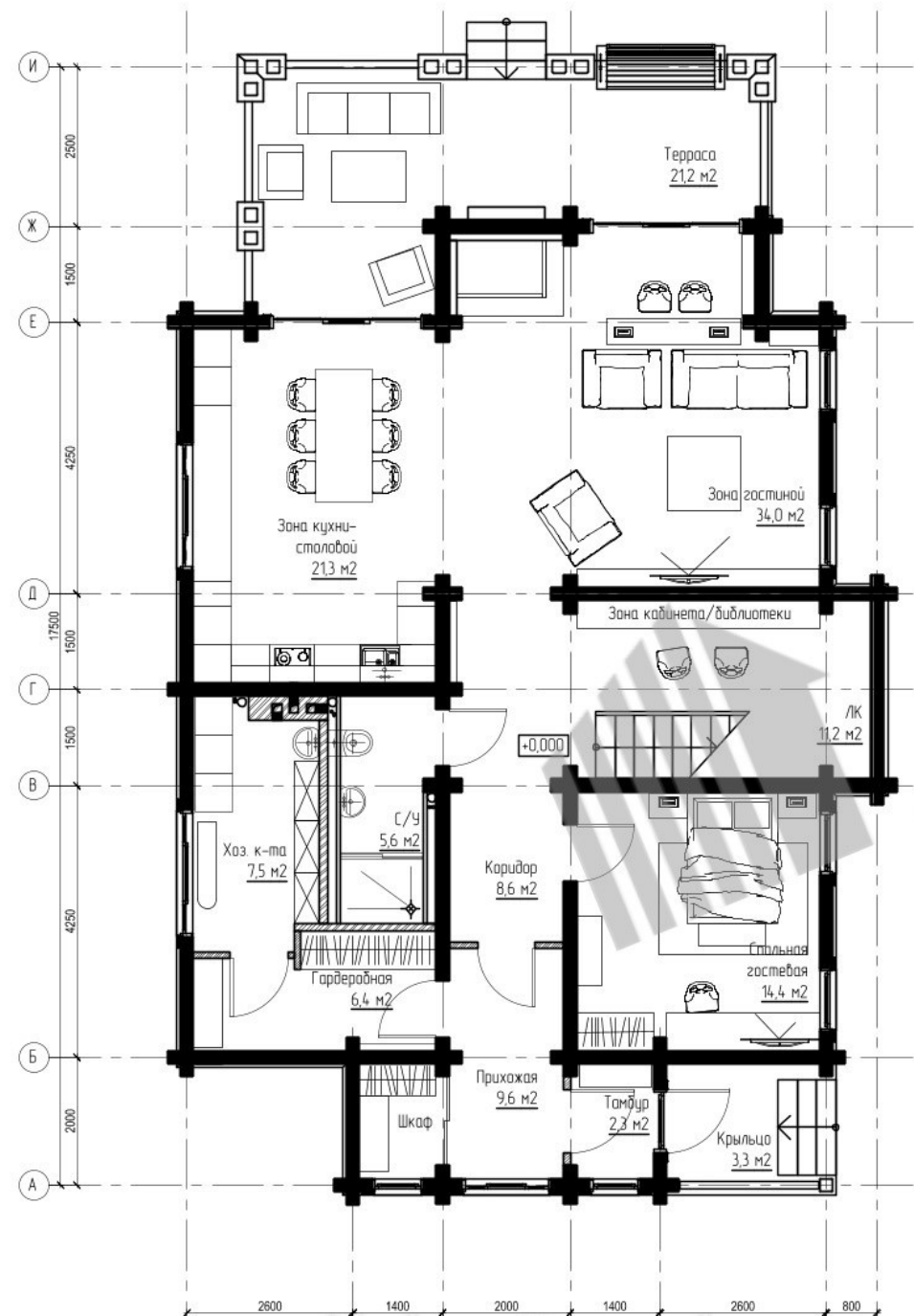
План 1 этажа М:100
