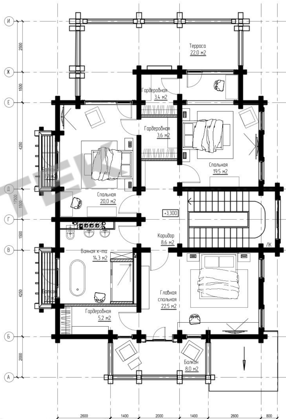
План 2 этажа М:100
